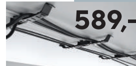
2 - křídla kabelová spona včetně kovové vodící lišty, 490 mm
